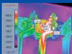
ÉCHAUFFEMENT D'UNE CONNEXION VISSÉE DE BARRE OMNIBUS.
